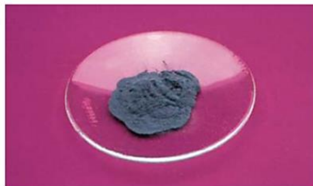
Tellurium (Te)
