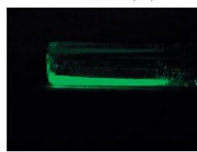
Radium (Ra)
