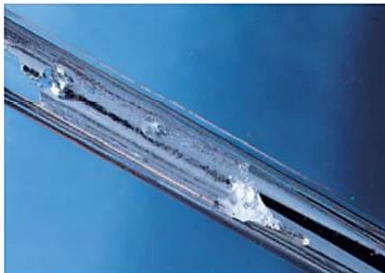
Rubidium (Rb)
