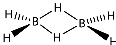
diborane ( B_2H_6 )
