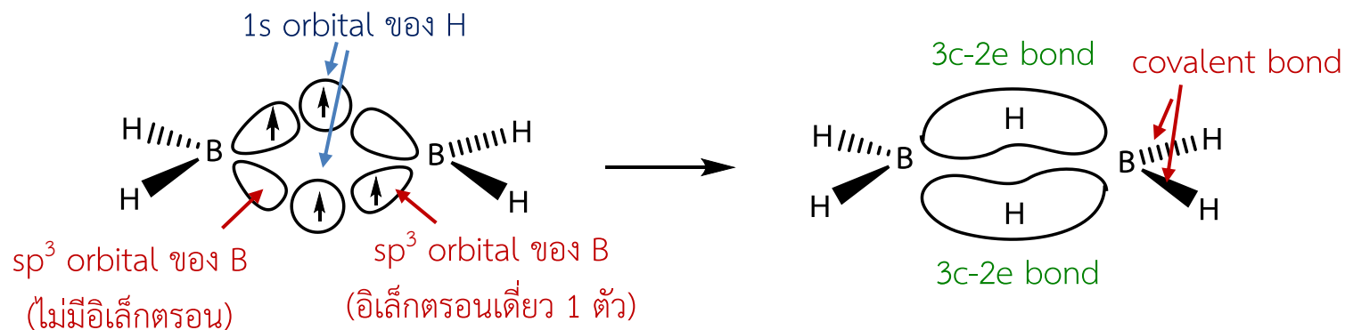
diborane ( B_2H_6 )
