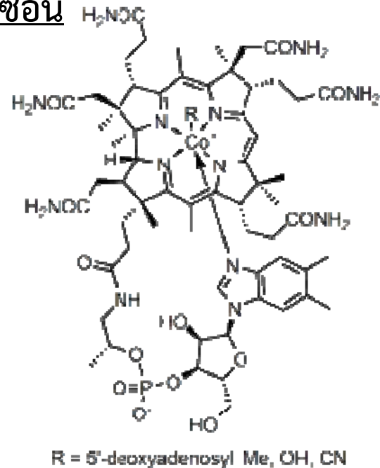
Vitamin B-12
